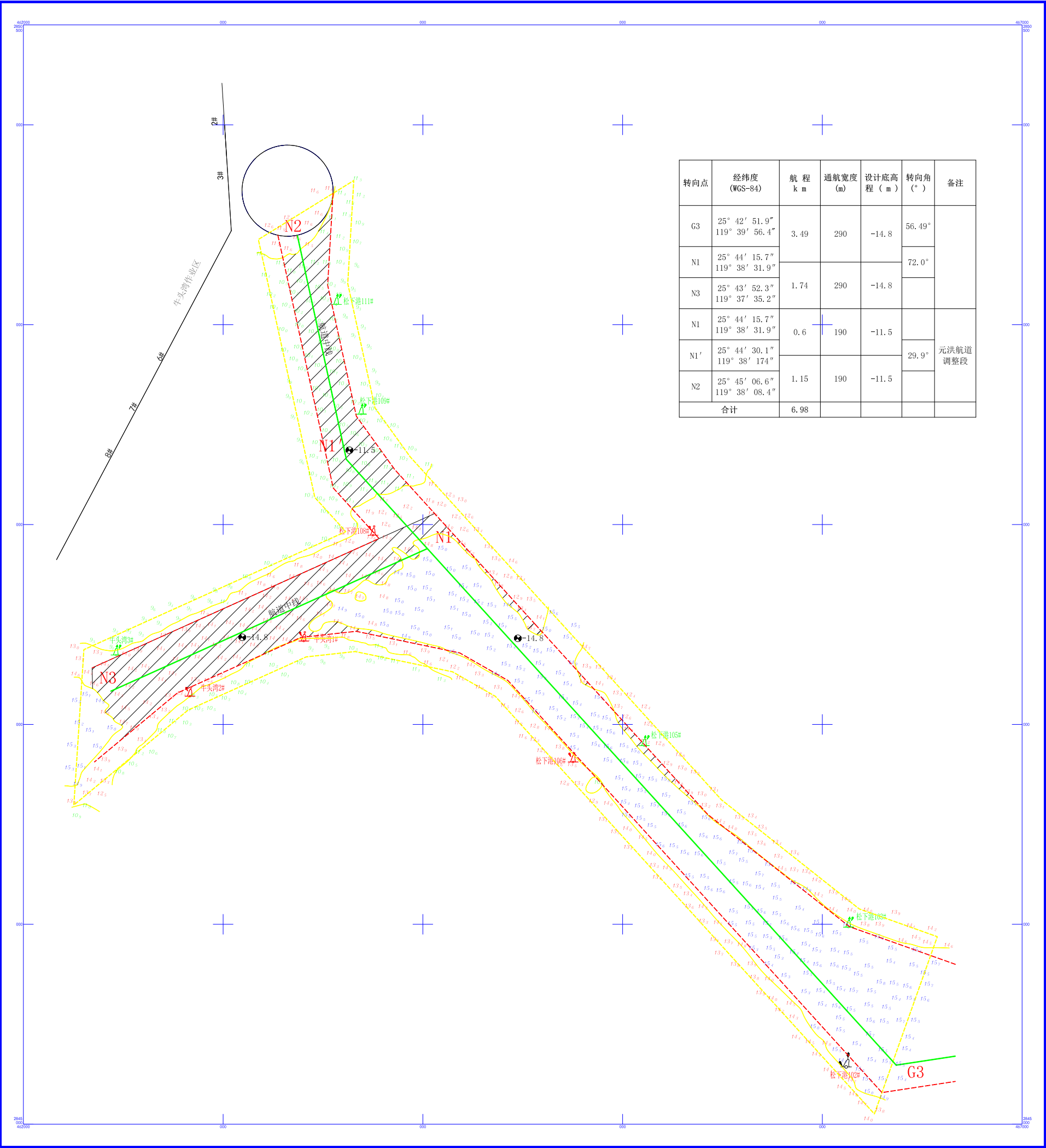
福州港福清湾深水航道二期工程水深图
